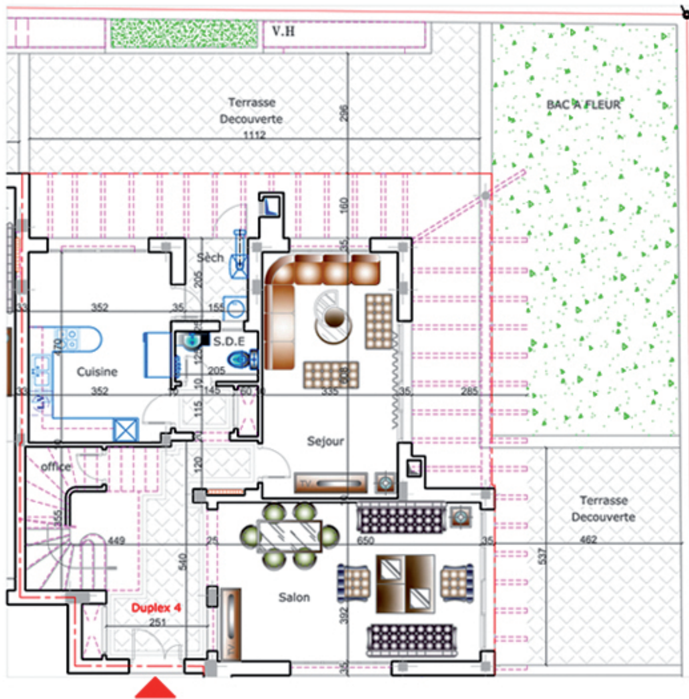
PLAN REZ DE CHAUSSEE
